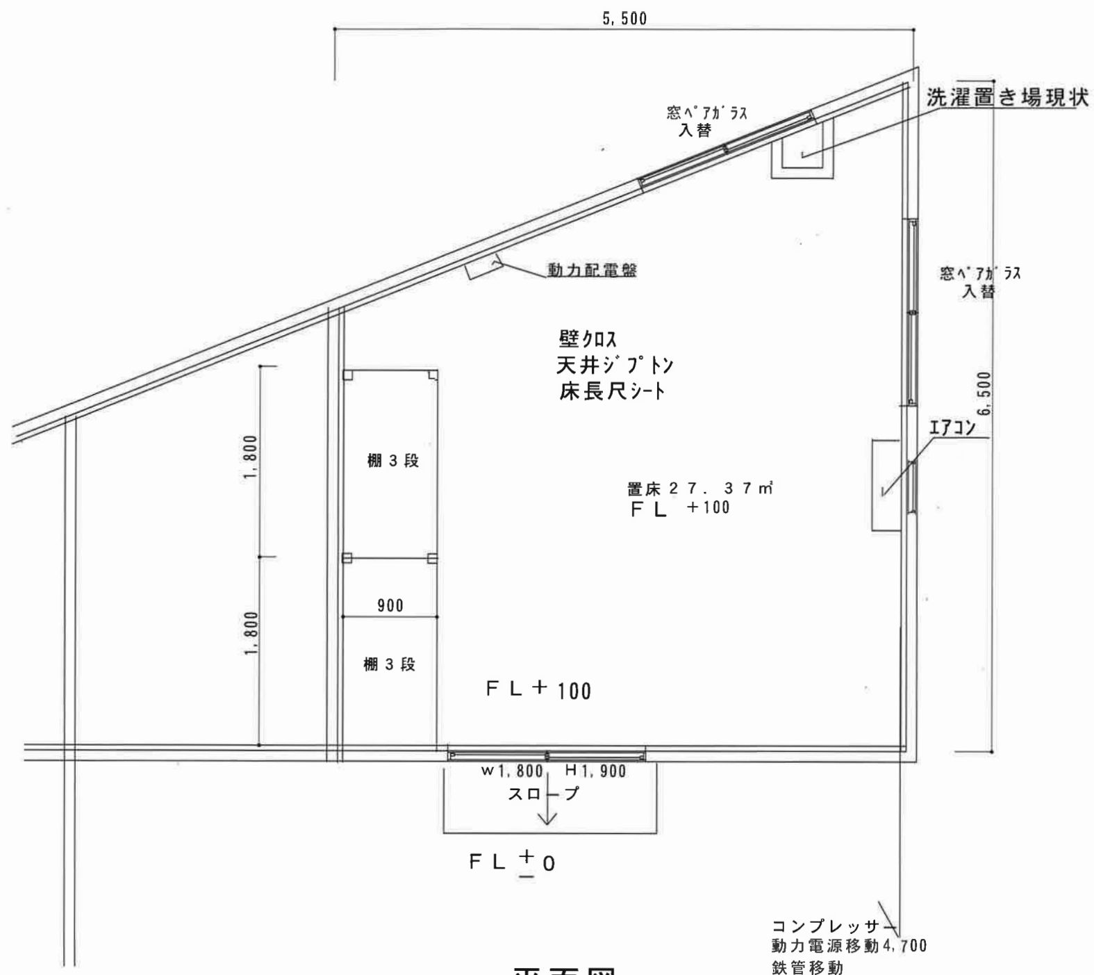
平面図
